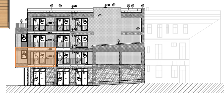
Pohľad JUŽNÝ
